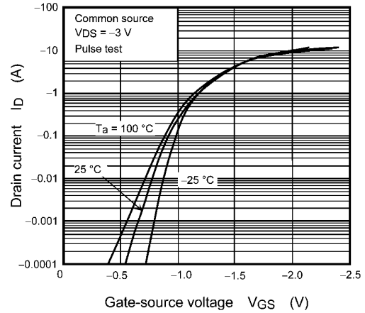
Fig. 8.2 I_D - V_{GS}
