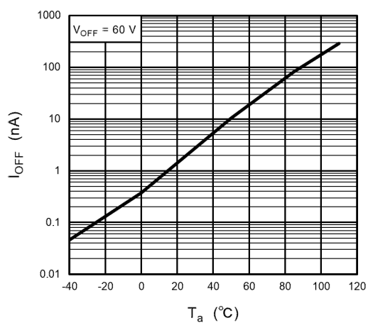
Fig. 14.1.9 I_{OFF} - T_a
