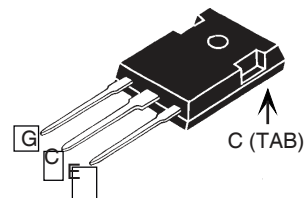
TO-247 (IXGH)
