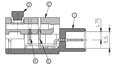
SECT A-A
