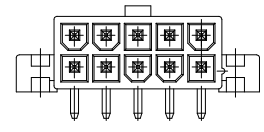
CKT. SIZE 10
