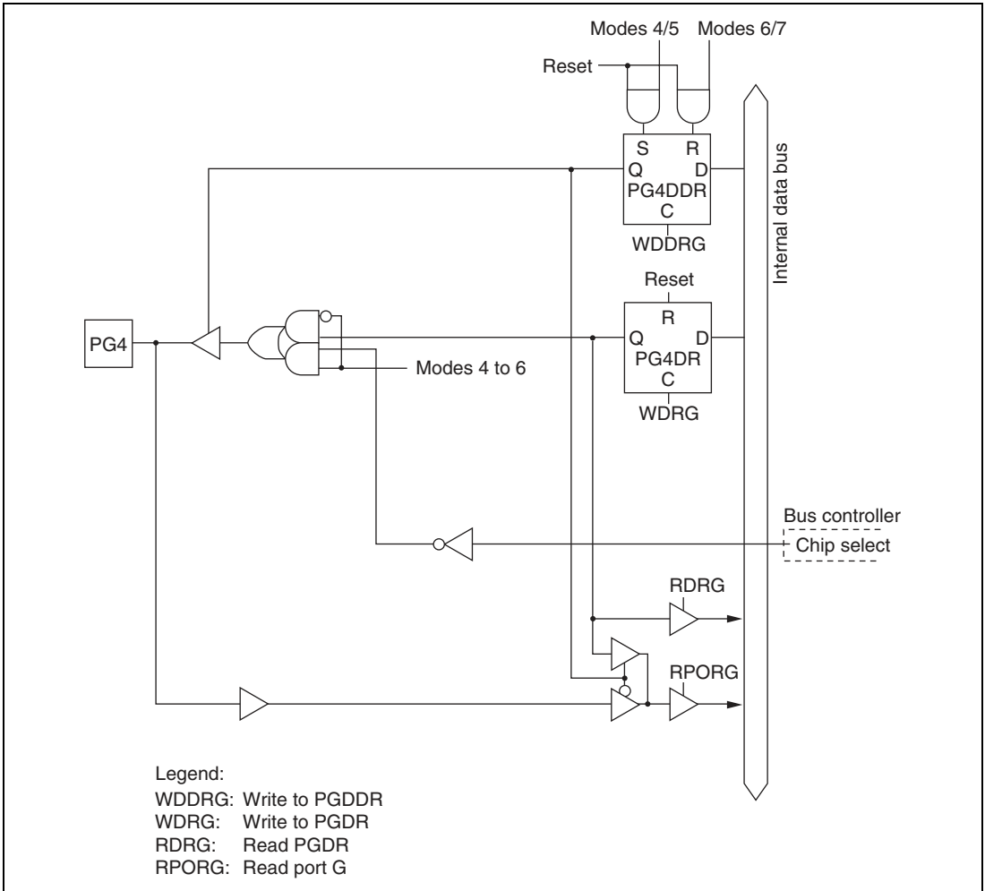
Figure C.24 (d) Port G Block Diagram (Pin PG4)
