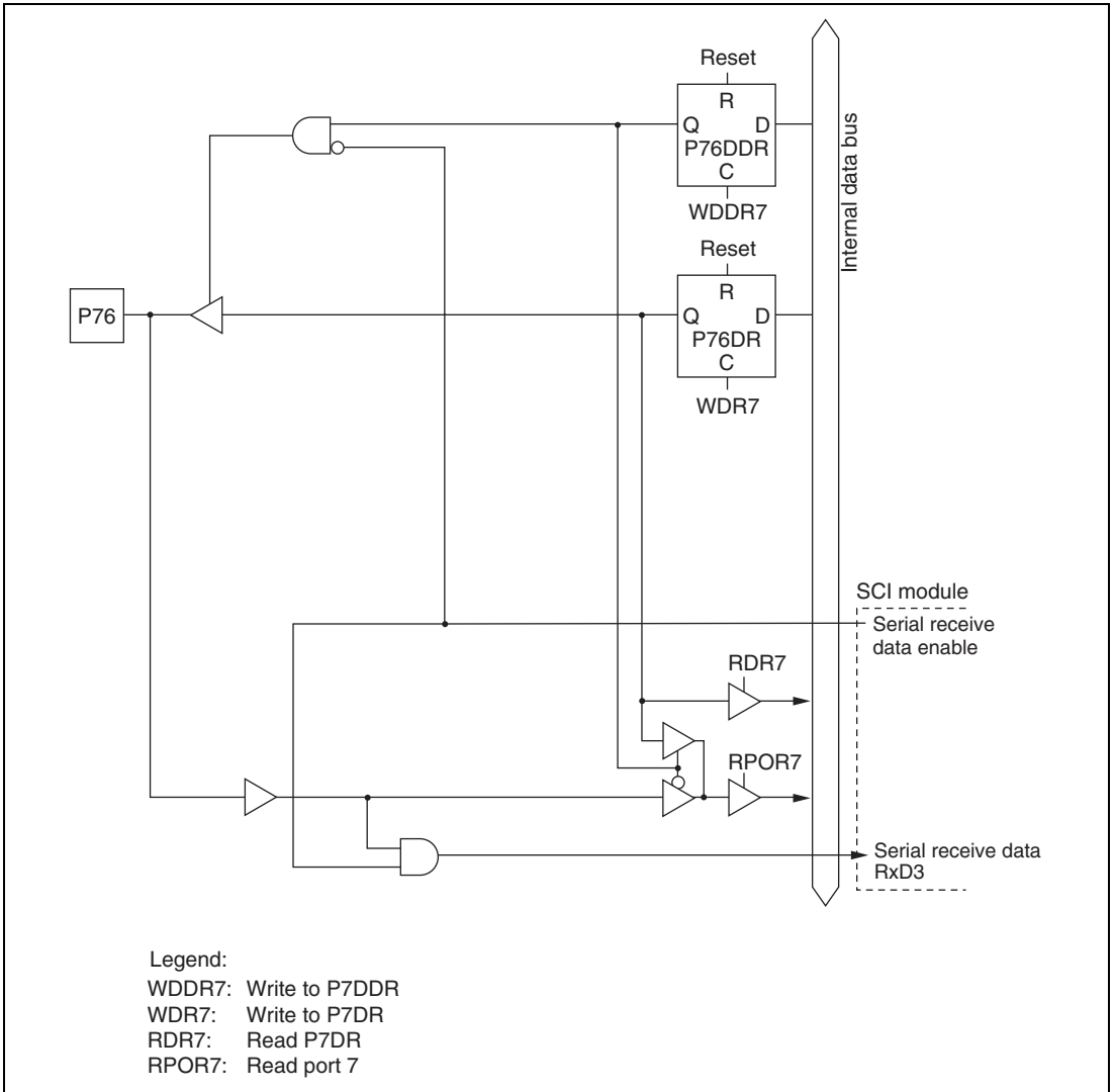
Figure C.16 (d) Port 7 Block Diagram (Pin P76)
