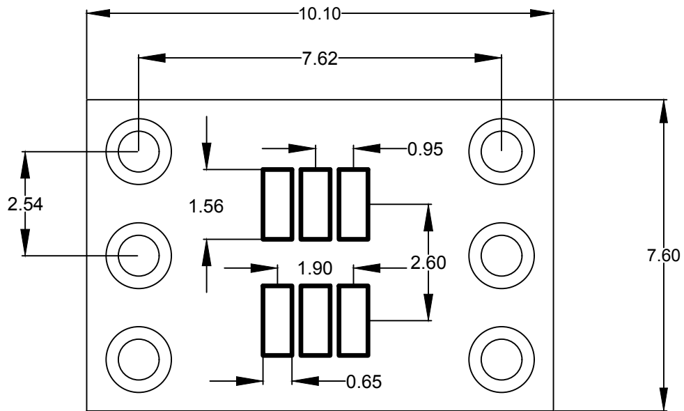
Front: SOT23-6
