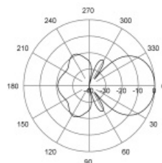
E-Plane | 832 MHz
