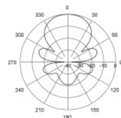
H-Plane | 832 MHz
