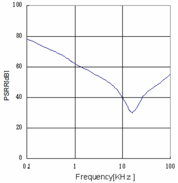
Fig. 32 PSRR (Io=0mA)
