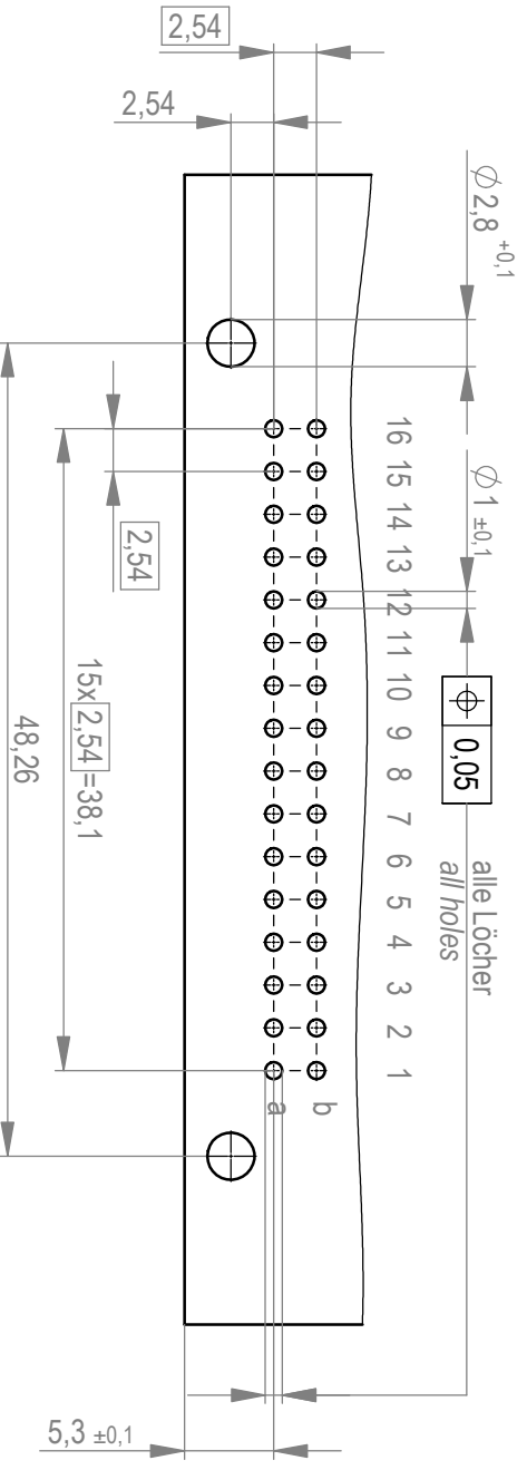
Leiterplatten-Lochbild / PCB drillhole pattern
