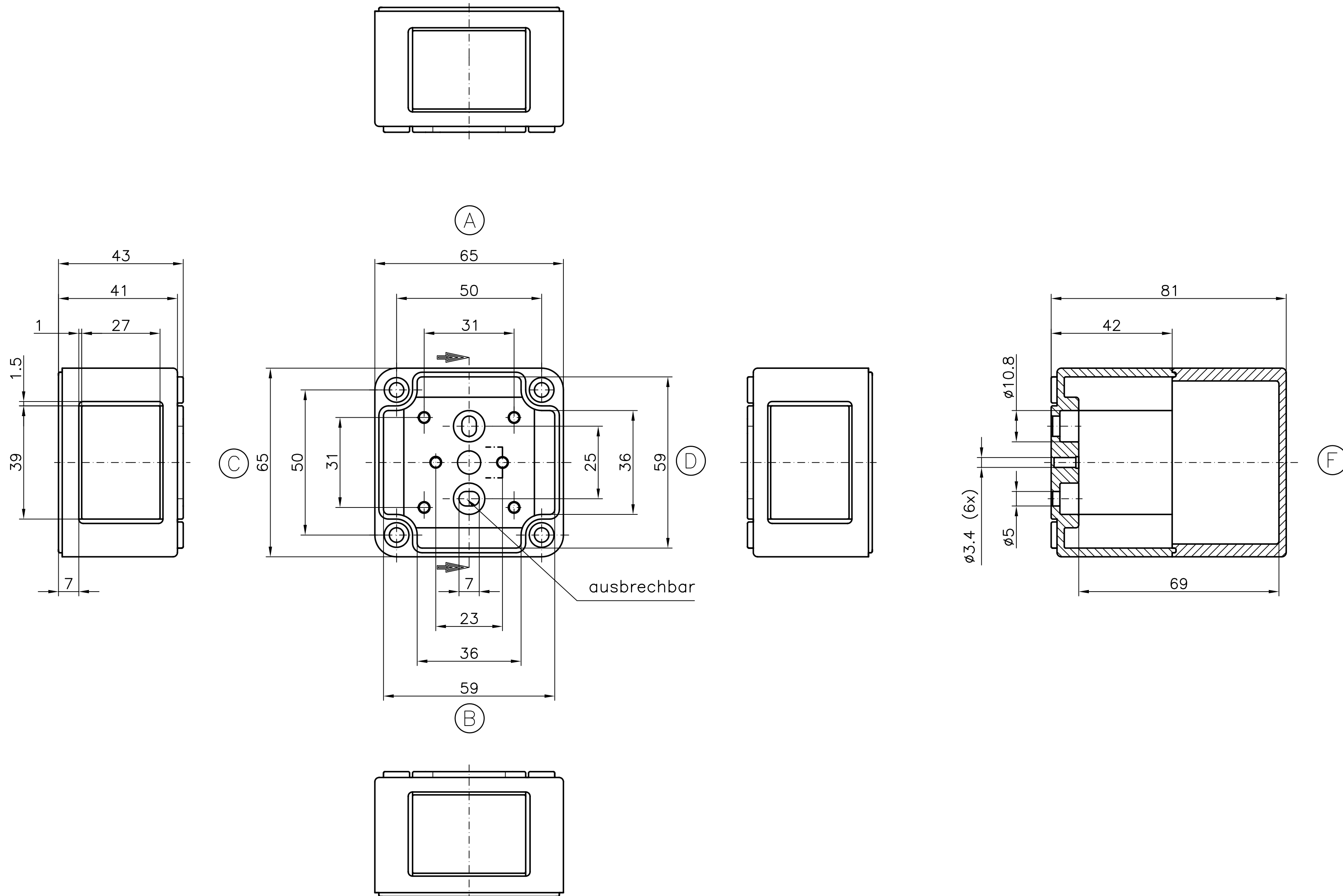
Kompaktgehäuse ECO 01-8 Bestell-Nr. 60.070721
