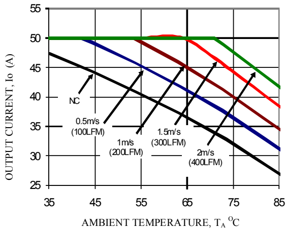
V_o=1.8V , V_{in}=12V
