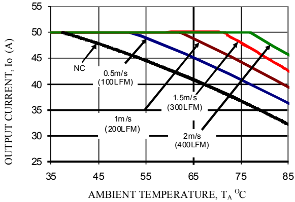
V_o=0.7V , V_{in}=12V
