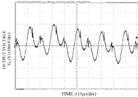
Vo=1.8V, Ta=25°C, Vin=12V, Io = Io,max
