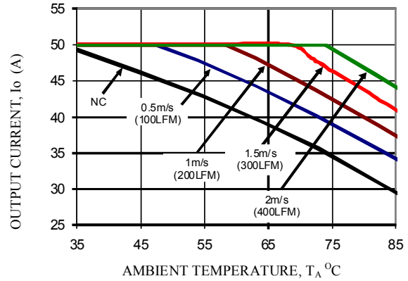
V_o=1.2V , V_{in}=12V
