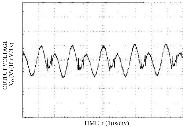
Vo=0.7V, Ta=25°C, Vin=12V, Io = Io,max
