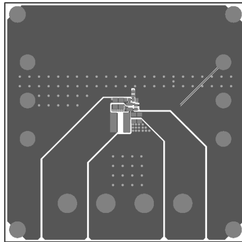
Figure 4—Top Layer
