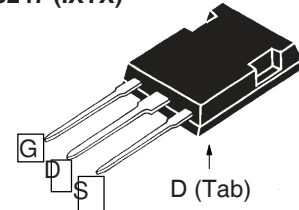
PLUS247 (IXTX)
