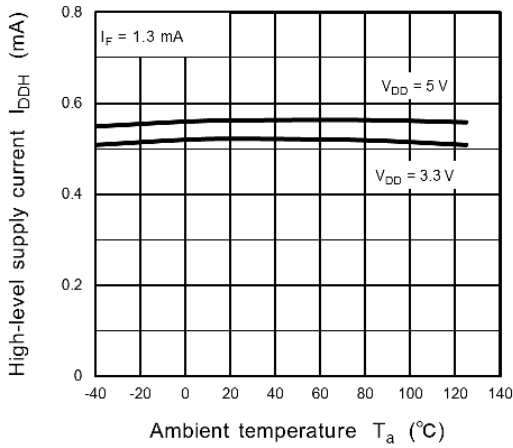
Fig. 12.2.7 I_{DDH} - T_a
