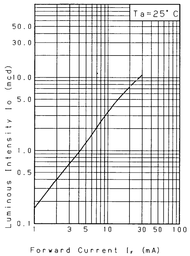
I_o - I_F
