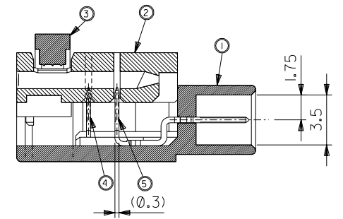
SECT A-A
