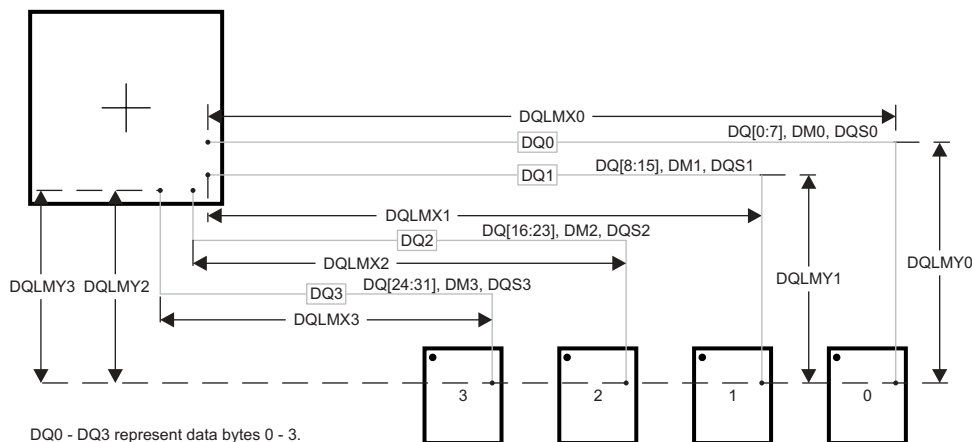
DQ0 - DQ3 represent data bytes 0 - 3.
