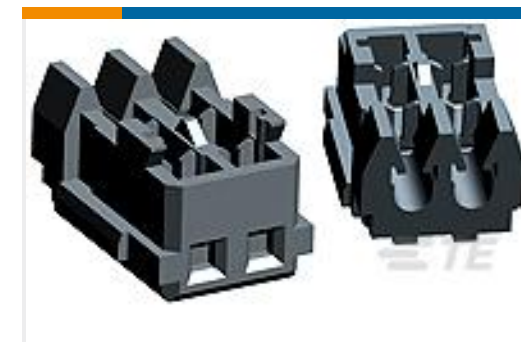
TE Part #353293-5 MINI CT MT REC ASSY 5P GRAY
