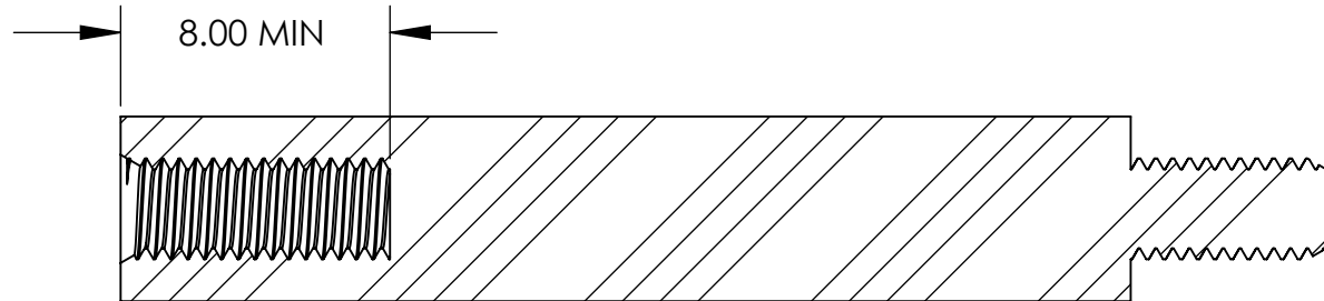
SECTION A-A SCALE 4 : 1
