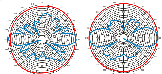
5.5 GHz H-Plane E-Plane 2.45 GHz
