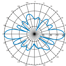
5.45 GHz E-Plane
