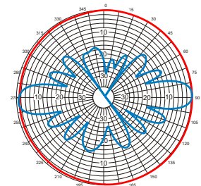
2.45 GHz ■ H-Plane ■ E-Plane
