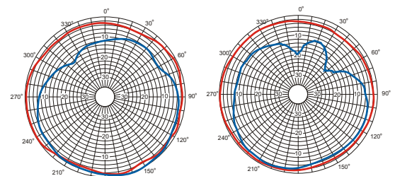
2.45 GHz ■ H-Plane ■ E-Plane 5.25 GHz
