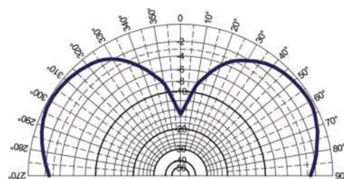
2.4 GHz ■ E-Plane
