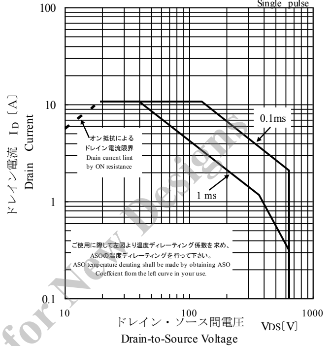
STR-Y6453 MOS FET A.S.O. 曲線 Ta=25°C curve
