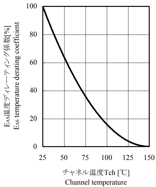
STR-Y6453 アバランシェ・エネルギー耐量 デレーティング曲線 Avalanche energy derating curve
