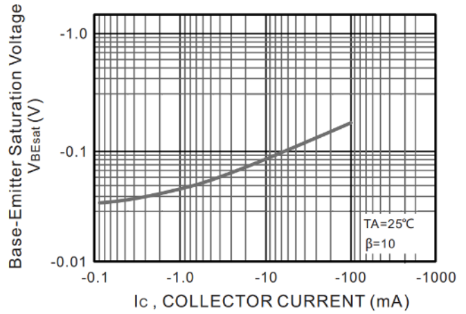
Fig.6 V_{CEsat}-I_c
