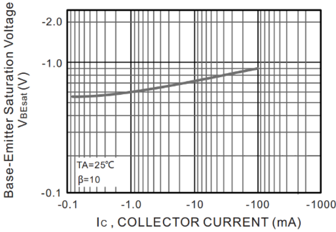
Fig.5 V_{BEsat}-I_c
