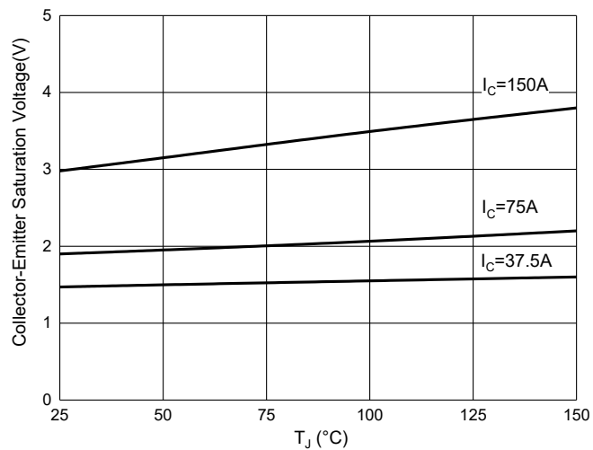
Fig. 4 - V_{CE(sat)} - T_J
