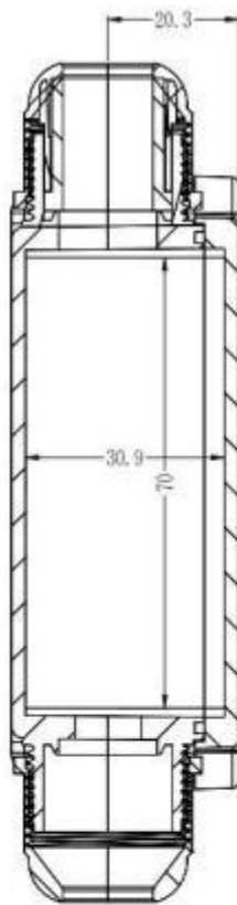
SECTION A-A
