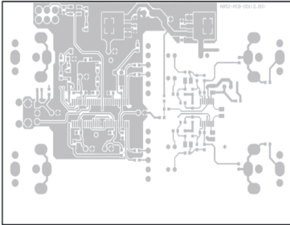
Figure 23. DRV603EVM PCB Top Layer
