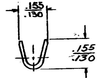
SECT A-A
