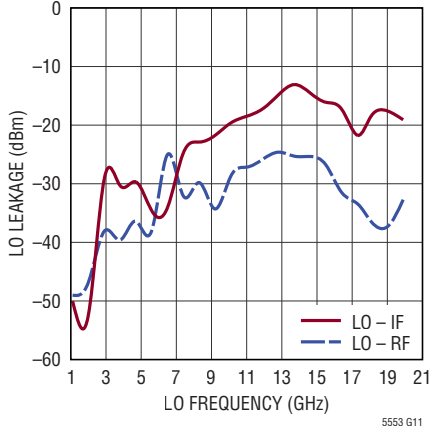
LO Leakage
