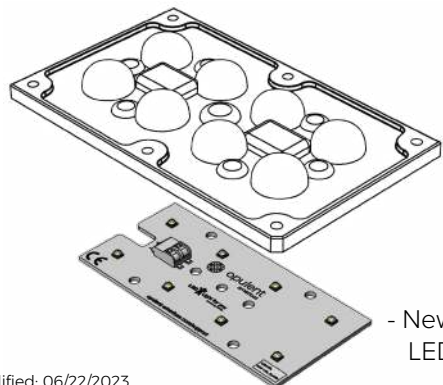
- Standard Khatod Optic, Nactus 4x2
