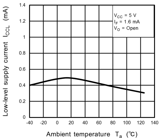
Fig. 12.2.5 I_{CCL} - T_a
