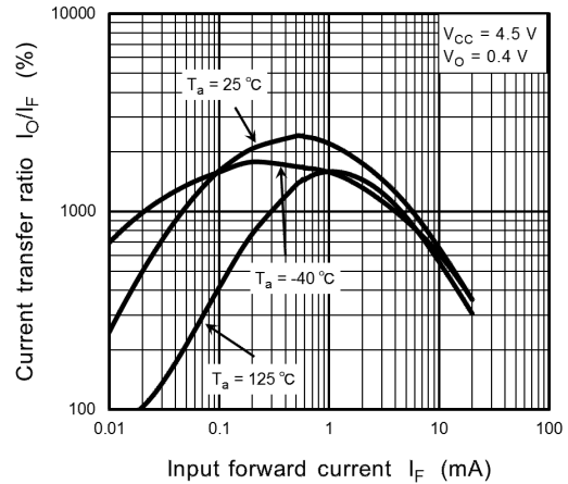
Fig. 12.2.8 I_O/I_F - I_F
