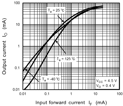
Fig. 12.2.7 I_O - I_F
