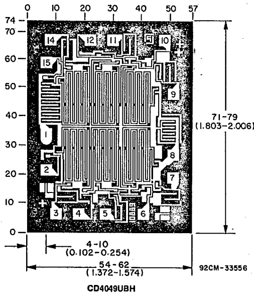
CD4049UBH
