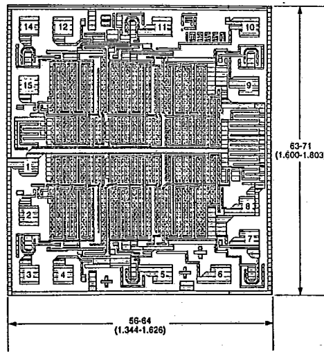
CD4050BH
