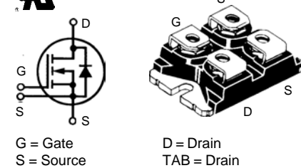
miniBLOC, SOT-227 B (IXFN)
