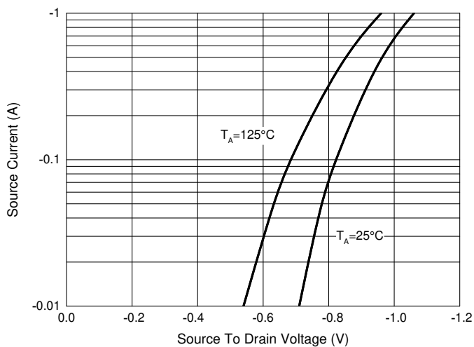
Fig. 5 - I_S - V_{SD}
