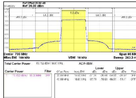
Figure 19. ACLR @700MHz, LTE20MHz 1 , -50dBc
