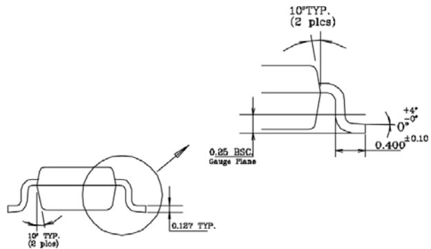
TSOT-23-5 (D5)
