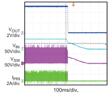
VIN Shutdown
