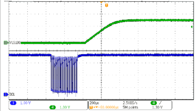
VBAT = 3.6 V
