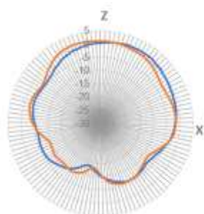
— 1575 MHz — 1602 MHz
