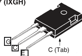
TO-247 (IXGH)
