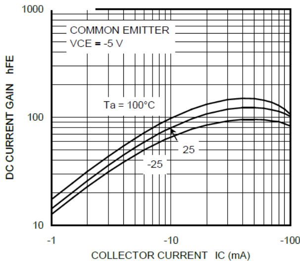
Fig. 10.11 RN2314 h_{FE} - I_C
