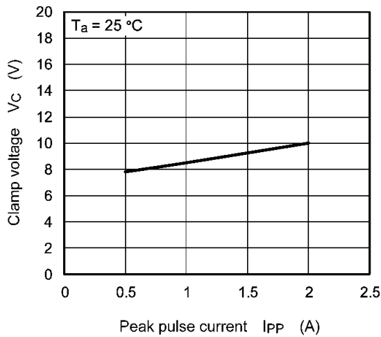
Fig. 6.3.1 V_C - I_{PP}
