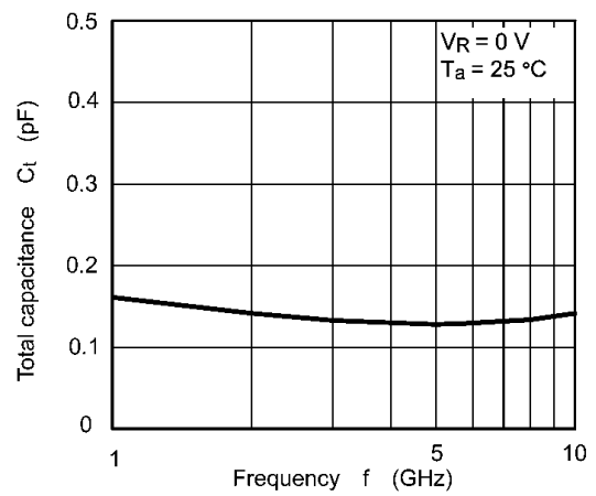
Fig. 9.4 C_t - f
