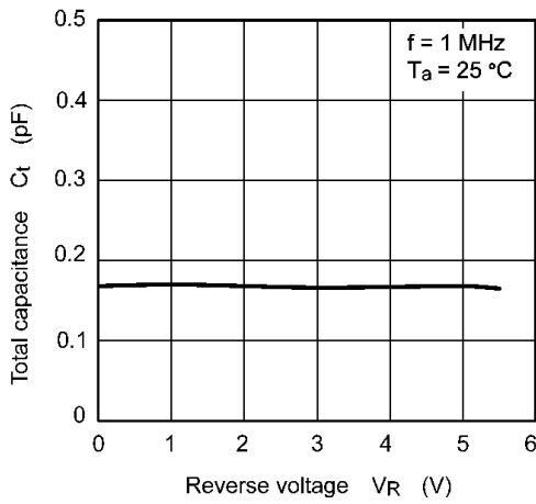
Fig. 9.3 C_t - V_R
