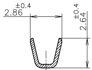
SECT A-A
