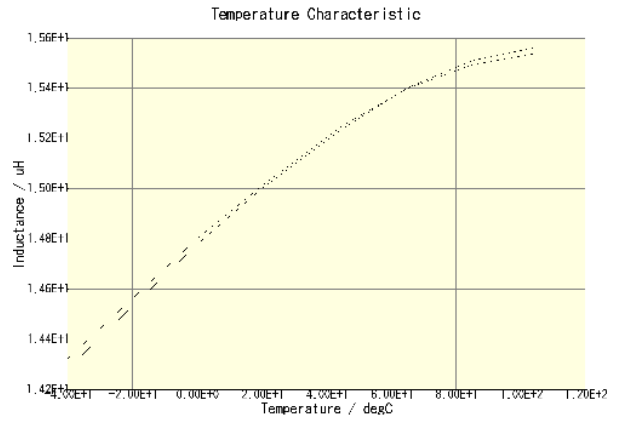
CLF12555T-150M-CA(DC = 0A)
