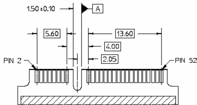
DETAIL Y
