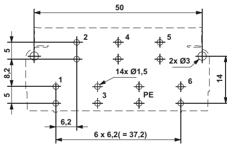
Drilling diagram: DC-...PCB-180
