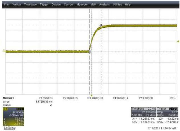
CH1:Vo (10 V/div)
