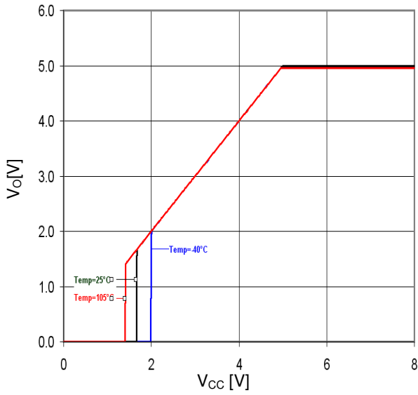
Figure 27. Vcc-Vo (Io=0mA)
