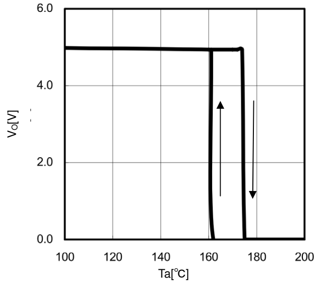
Figure 28. TSD (Io=0mA)
