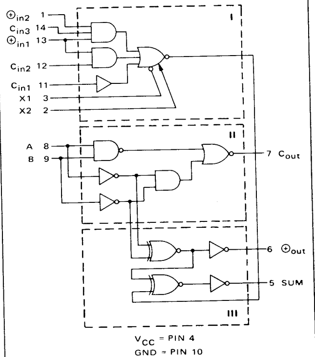
INDEPENDENT-CARRY FAST ADDER MC4330/4030, MC4331/4031
