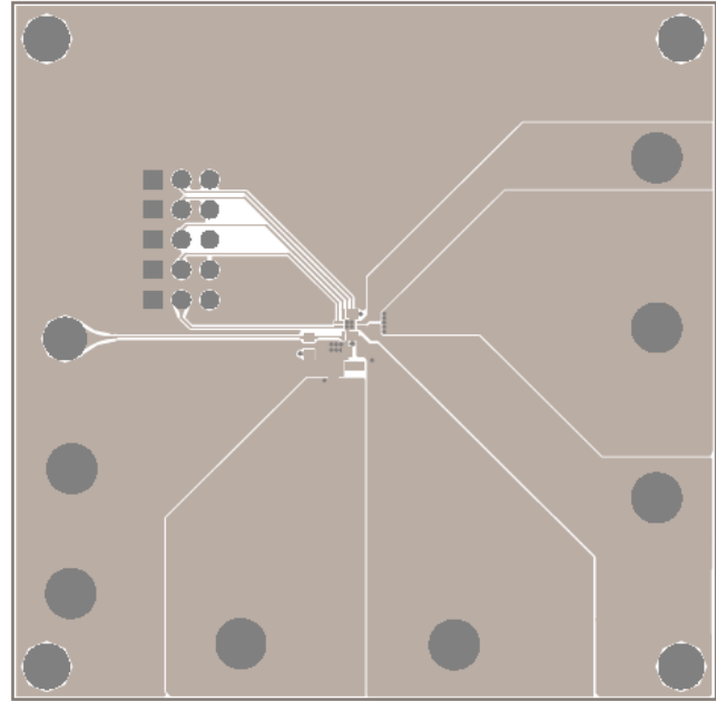
Figure 5—Top Layer
