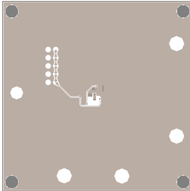
Figure 6—Bottom Layer
