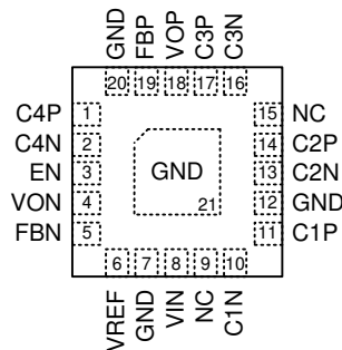
WQFN-20L 3x3
